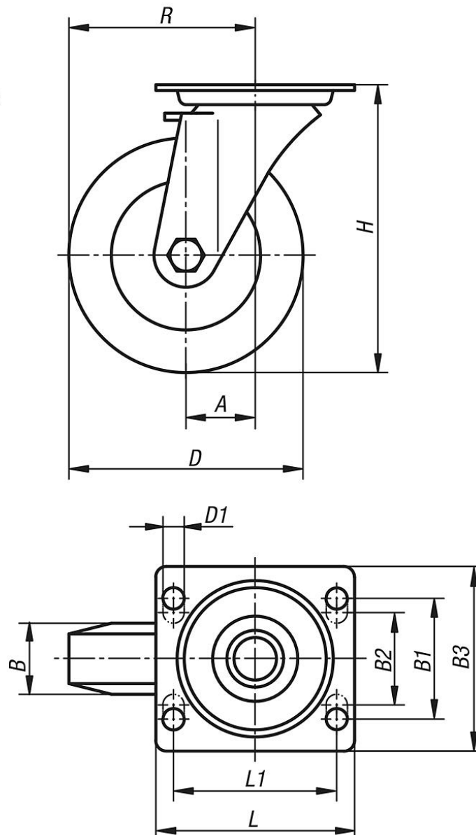
Lenkrolle
