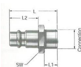
Nippel mit Außengewinde
