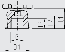
EN 837, Innengewinde
