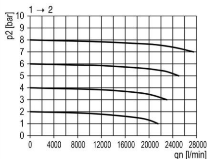
Durchflussdiagramm
