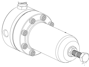
NeoFlow Pilot Ventil Baugruppe (montiert) mit schwarzer Feder, einstellbarer Druckbereich 1-8 bar
