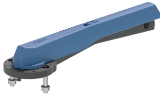
Handhebel zu Absperrklappe Typ 565 inklusive Schraubenset
